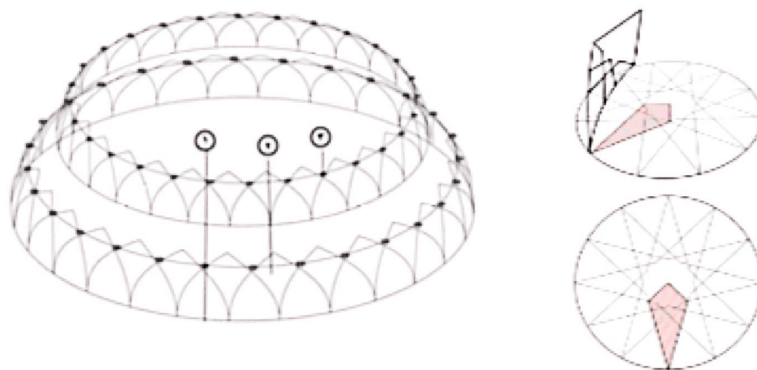
تحلیل سه بعدی گنبد یزدی بندی: ۱. ردیف های حلقوی افقی. ۲. واحدهای لوزی تکرار شونده. ۳. تخت های ستاره شکل.
