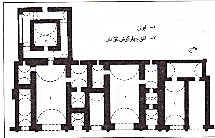
کاخ الحضر (بین النهرین یا میثرودان)، با ترکیبی از ایوان‌های ردیفی. در پشت یک ایوان فضای کوشک مانند دیده می‌شود.
