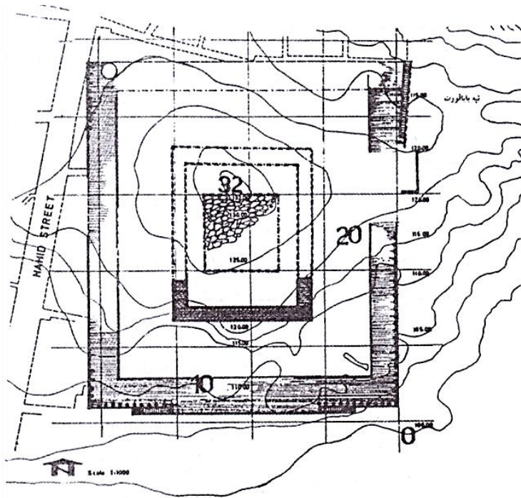
نقشه و پرسپکتیو بازسازی شده معبد آناهیتا در کنگاور
