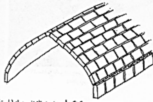
چگونگی اجرایی در طاق زنی چپله (راست) و استفاده از میل مهار در این شیوهی طاق زنی (چپ)
