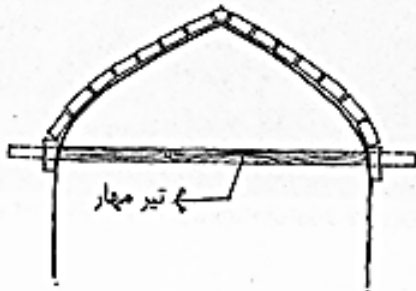
چگونگی اجرایی در طاق زنی چپله (راست) و استفاده از میل مهار در این شیوهی طاق زنی (چپ)
