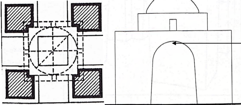
نگاره ۳۳-۳: نمای آتشکده
