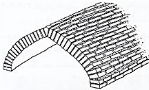
شیوه آجرچینی تاق به روش ایلامی
