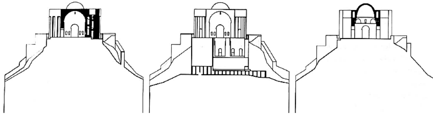
قلعه دختر فیروزآباد
