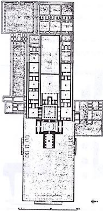
قصر شیرین، کاخ خسرو، نقشه مجموعه
