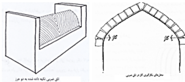
تاق ضربی تکمیل شده به دو جز
