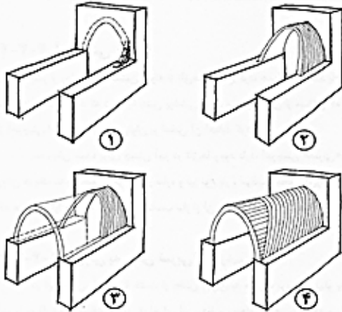
مراحل اجرای تاقی به روش ضربی
