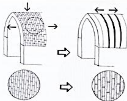
بربر شن تاق و وضعیت (جرها در دو حالت عالی (چپ) و بربر شده (راست)
