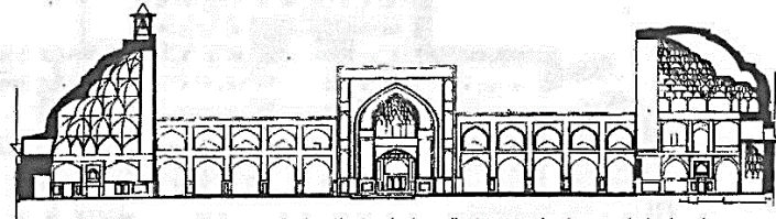
مسجد جامع اصفهان - برش غربی - شرقی و ایوان شمالی (صفه درویش)
