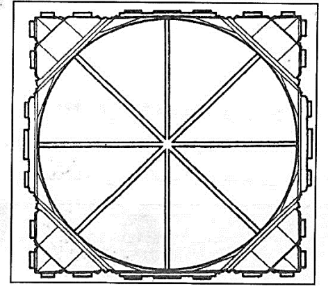
اصفهان - مسجد جامع، گنبد خواجه نظام‌الملک، ۴۷۳ هجری قمری، این گنبد دارای هشت ترک باربر است پوشش گنبد به روش ترکیب
