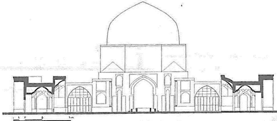
گلپایگان - برش عمودی ب-ب - نمای گنبدخانه و ایوان
