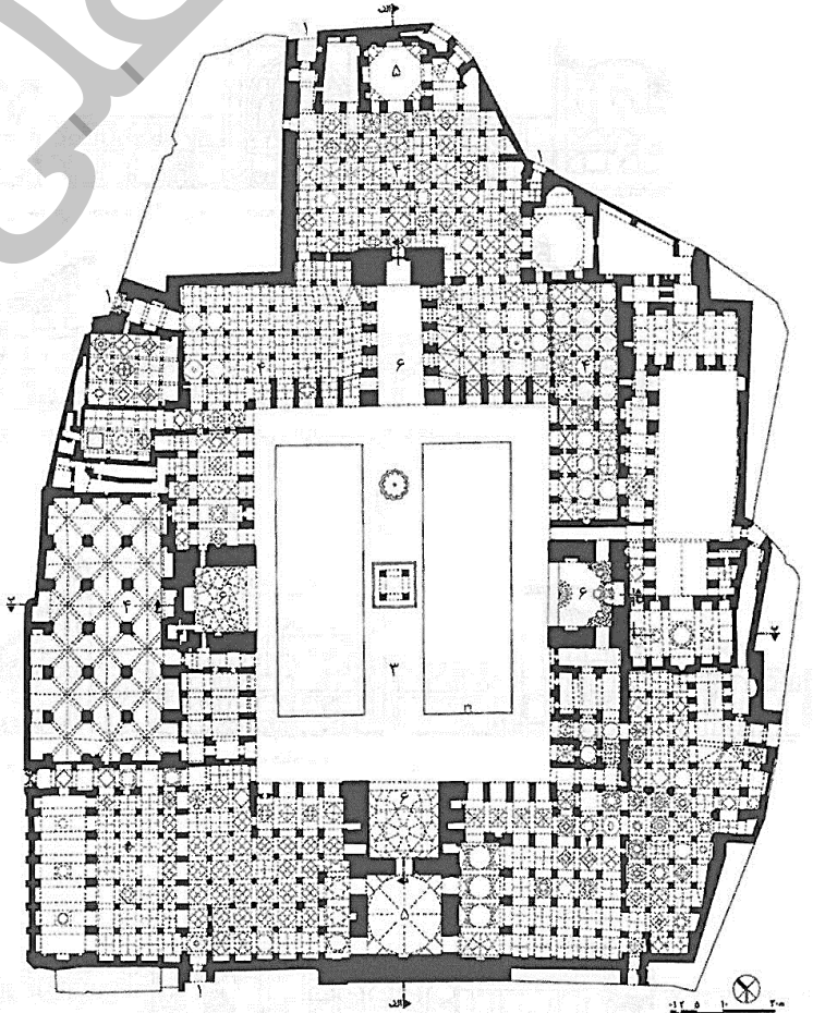
اصفهان - مسجد جامع، برش افقی طبقه اول
