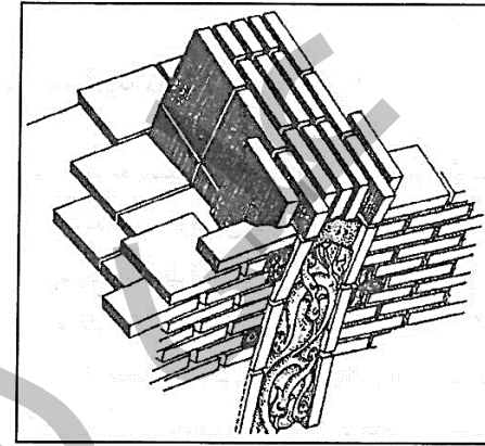
اصفهان - مسجد جامع، گنبد خواجه نظام‌الملک، ۴۷۳ هجری قمری، این گنبد دارای هشت ترک باربر است پوشش گنبد به روش ترکیب
