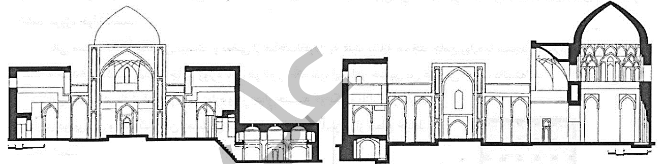
زواره - مسجد جامع - برش عمودی ب-ب
