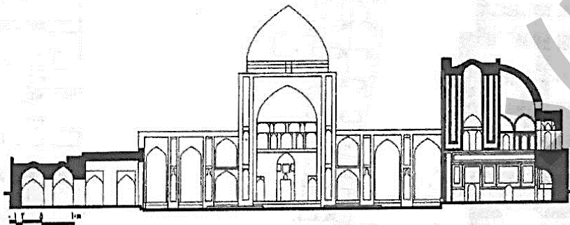
ساوه - مسجد جامع - برش عمودی الف-الف
