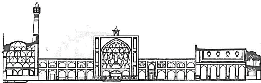
مسجد جامع اصفهان - برش شمالی - جنوبی و ایوان غربی (صفه استاد)
