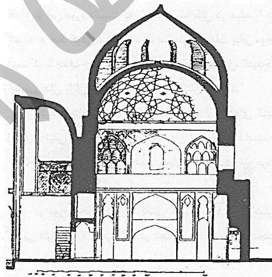
ساوه - مسجد جامع - مقطع گنبدخانه - آر تور پوپ
