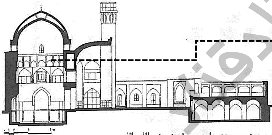
بروجرد - مسجد جامع - برش عمودی الف-الف
