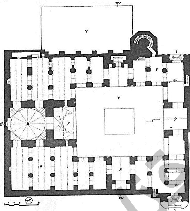
زواره - مسجد جامع - نقشه و برش افقی طبقه اول
