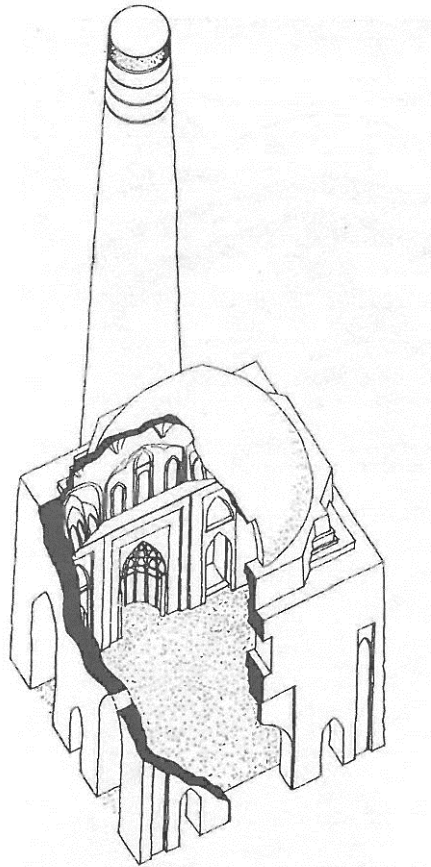
برسیان - مسجد جمعه - اسکیس
