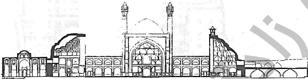
مسجد جامع اصفهان - برش غربی - شرقی و ایوان جنوبی (صفه صاحب)
