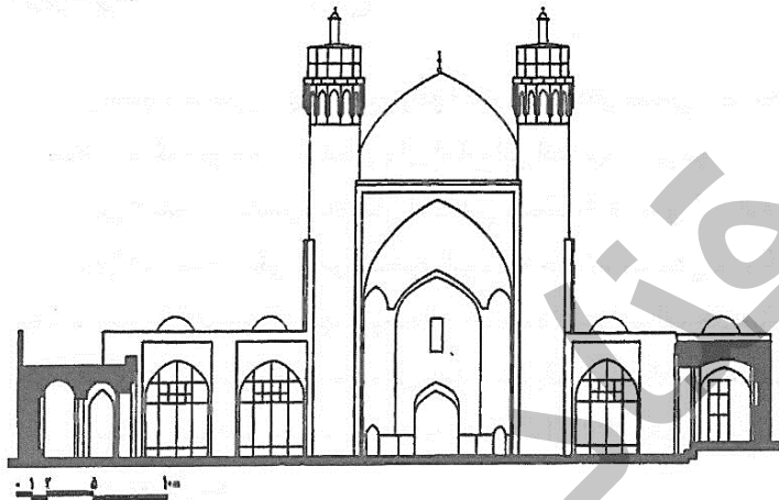
بروجرد - مسجد جامع - برش عمودی ب-ب
