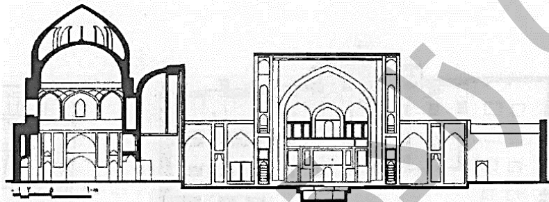
ساوه - مسجد جامع - برش عمودی ب-ب
