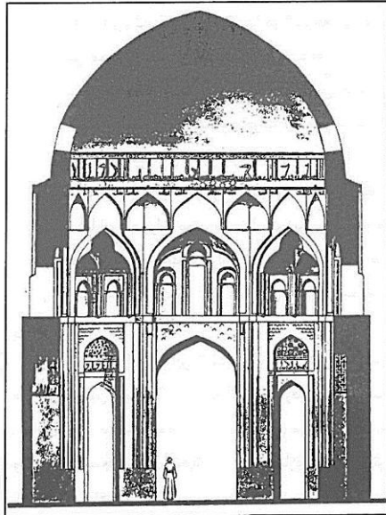
اصفهان - مسجد جامع، گنبد تاج‌الملک، ۴۸۱ هجری قمری، یکی از خوش‌تناسب‌ترین گنبدهای ایرانی (از بوب)
