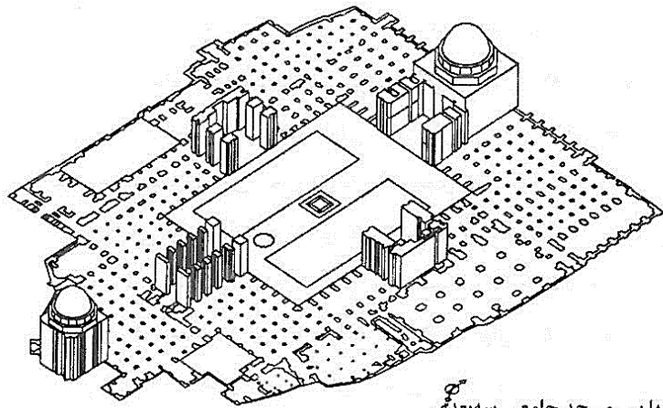
اصفهان - مسجد جامع - سه‌بعدی مجموعه نخستین تغییرات از نقشه شبستانی به گنبدخانه‌ای و چند ایوانی
