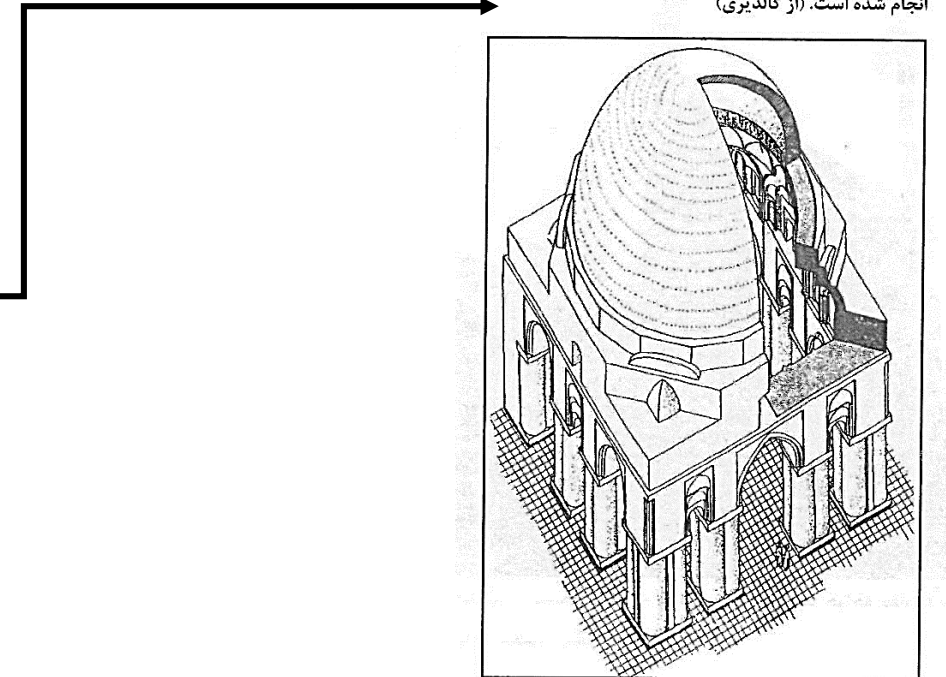
اصفهان - مسجد جامع، تصویر سه‌بعدی گنبد خواجه نظام‌الملک
