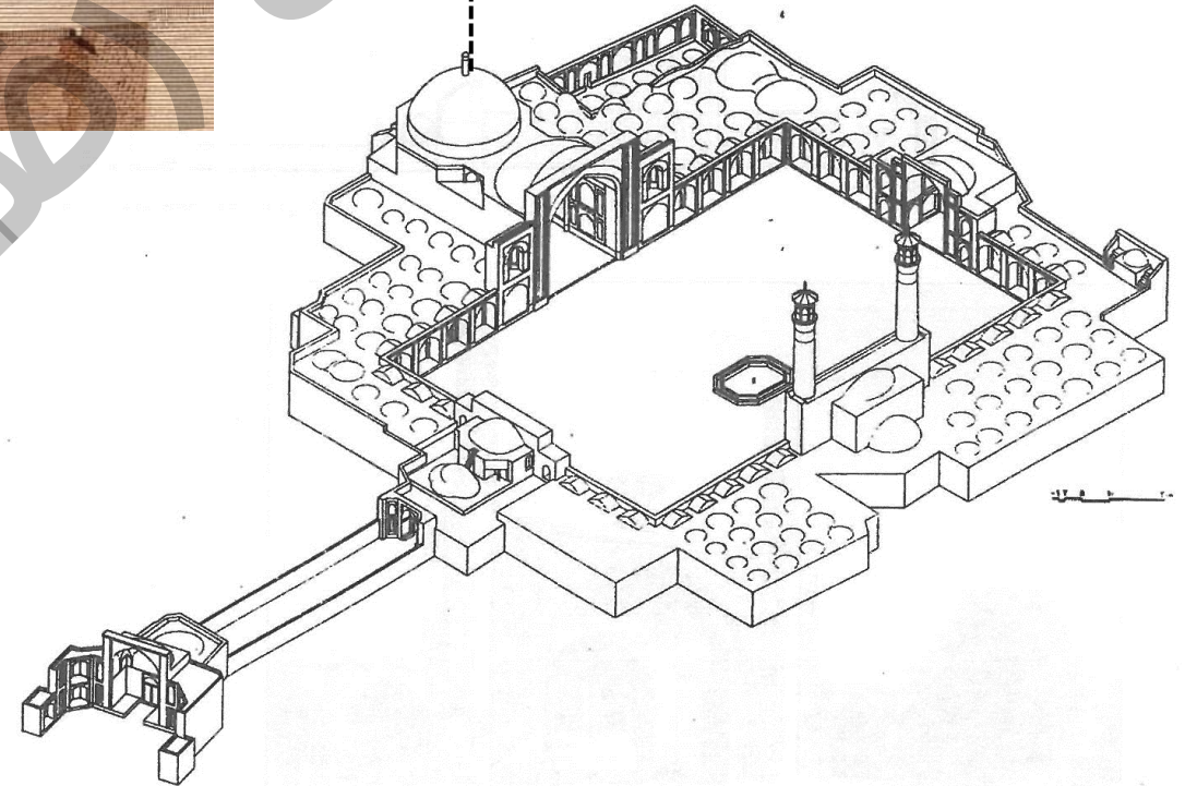
قزوین - مسجد جامع - تصویر سه بعدی
