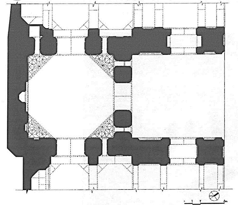
گلپایگان - مسجد جامع - برش افقی گنبدخانه و ایوان
