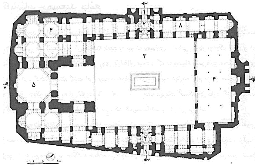
گلپایگان - برش افقی مسجد جامع
