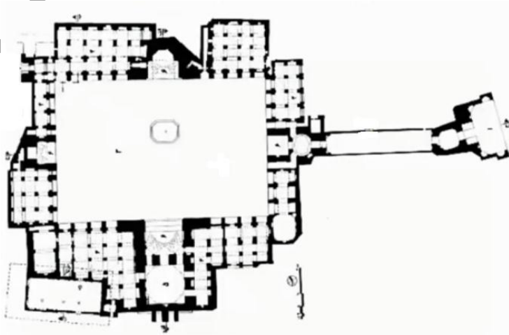
پلان و سه بعدی مسجد جامع قزوین
