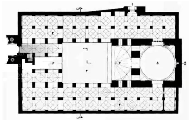
پلان و برش مسجد جامع اشترجان
