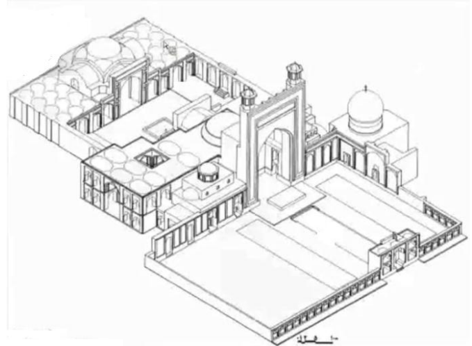
سه بعدی و پلان مجموعه احمد جام
